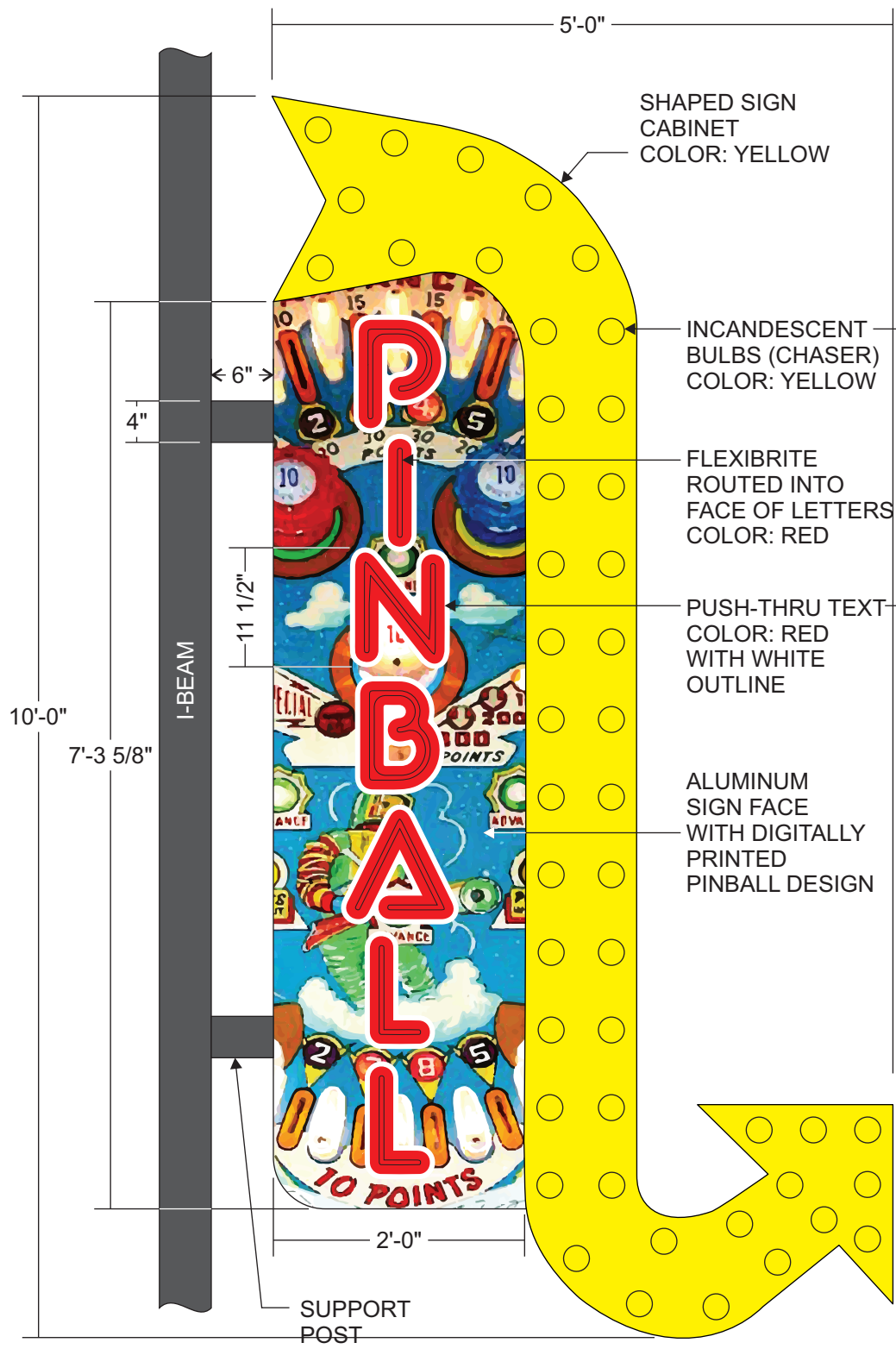
SIDE A SCALE: 3/4" = 1'
